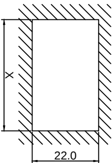
安裝開孔尺寸 PANEL HOLE SIZE
